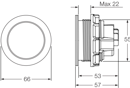
Pneumatisk spolknapp
