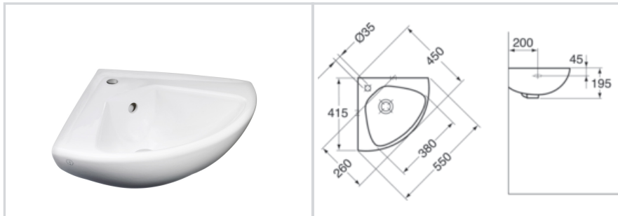
Måttolerans porslin 2%
