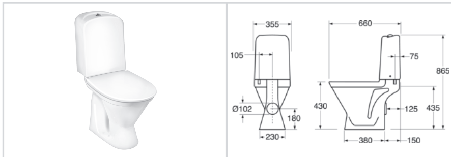
3510 Nordic 3 WC med dolt P-lås för golvmontage Måttolerans porslin 2%
