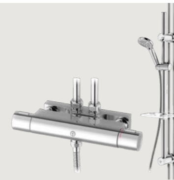
Duschpaket Nya Nautic 2.1 – termostat RSK 8350182 Inkl. duschset, vaska, energiklass A, blandarfäste 160/40 c-c
