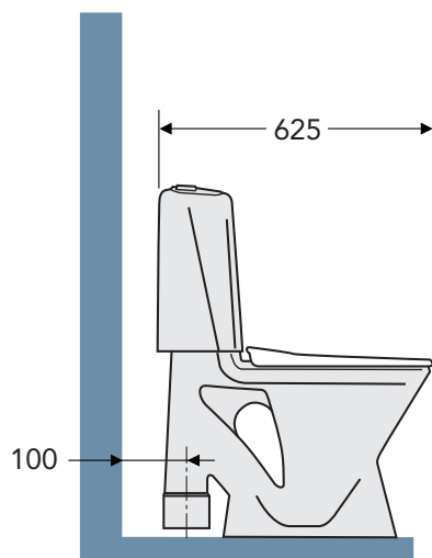
UZ GRĪDAS UZSTĀDĪTS TUALETES PODS
