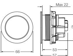
Mehānisks, augšpusē uzstādīts vadības panelis, Duo, pulēts hroms, plastmasa.
