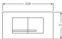
Mehānisks, augšpusē uzstādīts vadības panelis, Duo, pulēts hroms, plastmasa.
