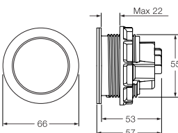
Mehānisks, augšpusē uzstādīts vadības panelis, Duo, pulēts hroms, plastmasa.
