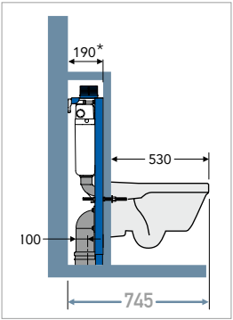
KORVATTU SEINÄÄN ASENNETTAVALLA WC- ISTUIMELLA, JOSSA ON TRIOMONT-ASENNUSTELINE
