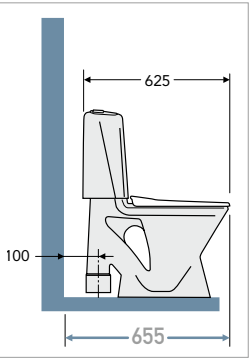
LATTIAAN ASENNETTU WC-ISTUIN
