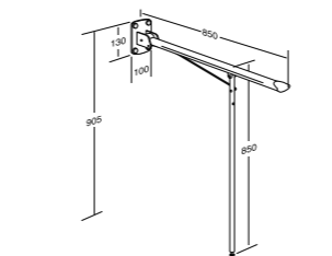
1712 käsinoja tukijalalla, pit. ja kork. 850 mm
