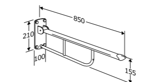
1711 käsinoja, pituus 850 mm
