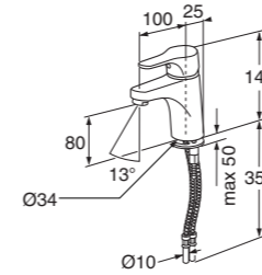
Nautic-pesuallashana Ilman vipupohjajaventiiliä
