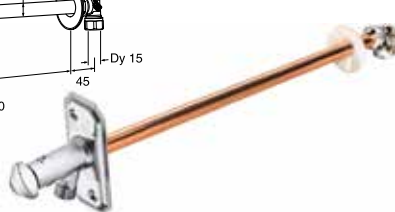
Udendørshane med typegodkendt kontraventil og greb, selvtømmende Vægtykkelse max 30–400 mm
