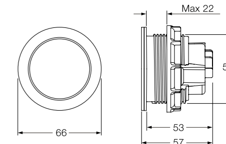
Pneumatisk spyleknapp
