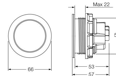
Pneumatisk skylleknop
